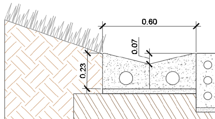
Figura 3-2 Detalle de cunetas
