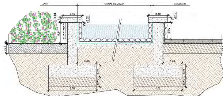
Figura 4-4. Esquema canal.
