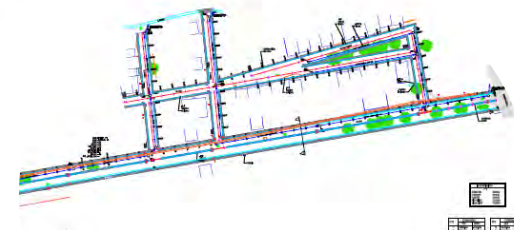
Propuesta de diseño de la red de acueducto y alcantarillado
