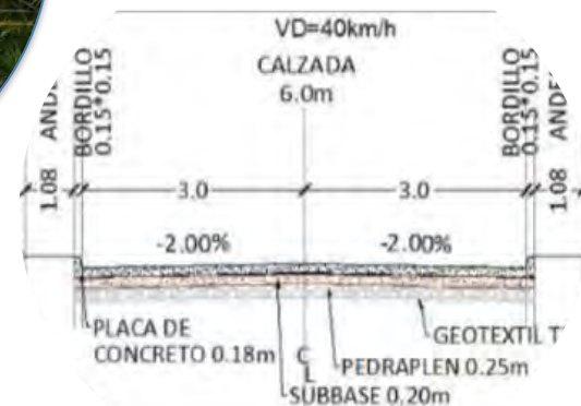
Sección Transversal Típica
