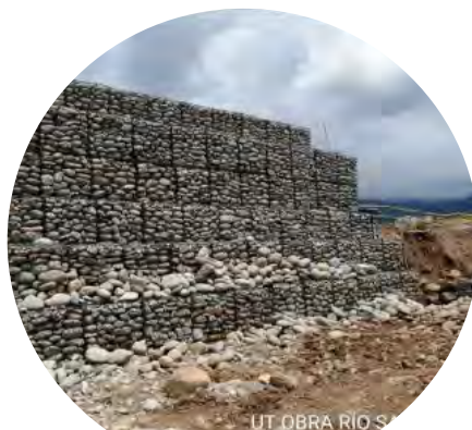
Construcción Azud 13
