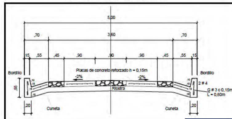
Detalle de Placa Huella
