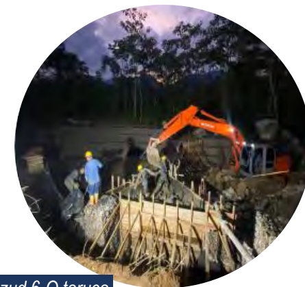
Fundición cuerpo Azud 6-Q taruca.
