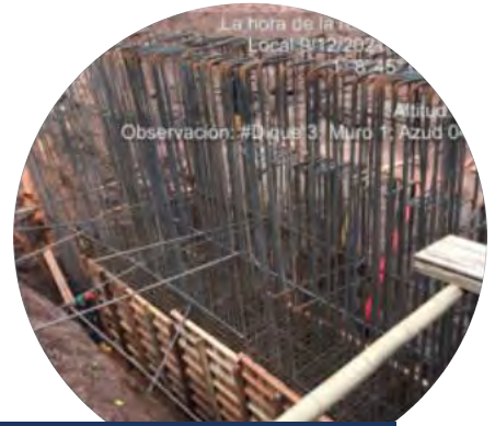
Instalación de acero y armado de formaleta para Dique 3 abierto
