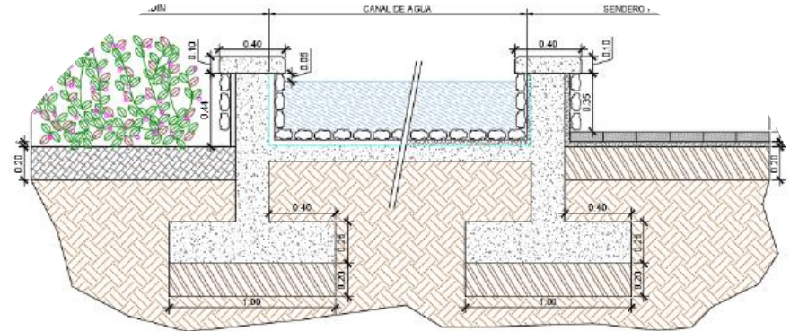
Figura 4-4. Esquema canal.
