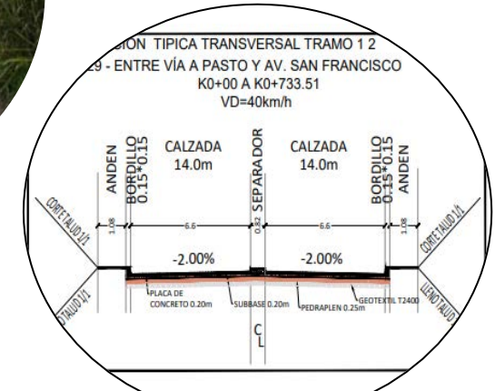
Sección transversal de la estructura de pavimento
