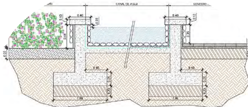
Figura 4-4. Esquema canal.
