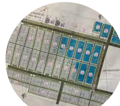
Avance movimiento de tierras
