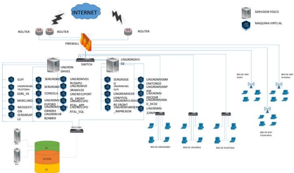
Ilustración 3. Diagrama de red sede principal UNGRD
