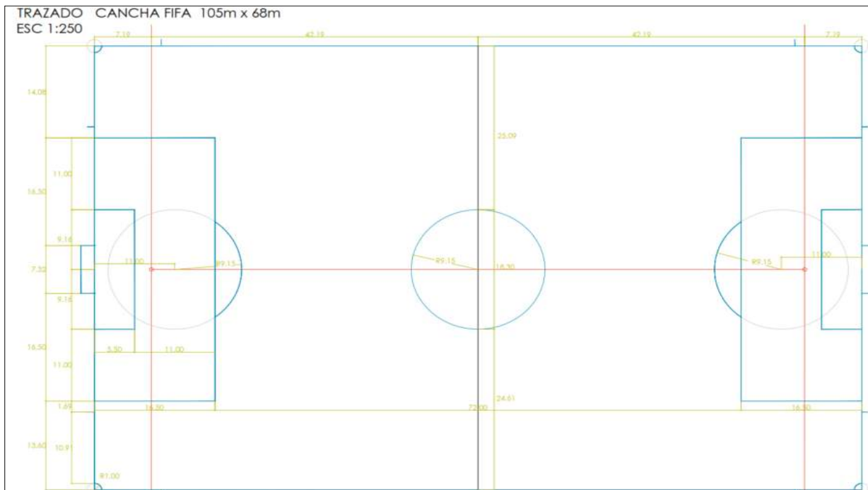
Ilustración 5. Planta General Cancha de Fútbol Estadio Marino Klinger
