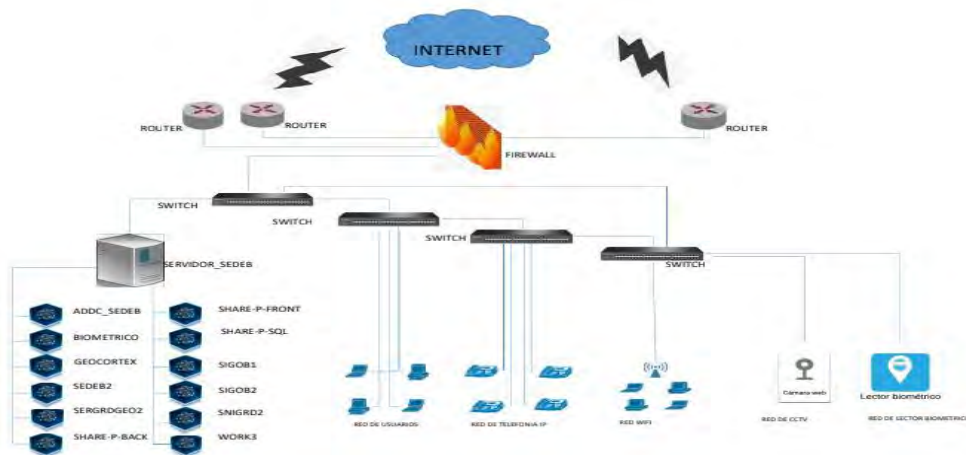
Ilustración 4. Diagrama de red Sede B UNGRD
